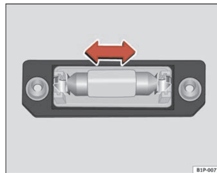
Abb. 201 Kennzeichenbeleuchtung
