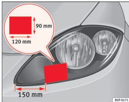
Abb. 157 Linker Scheinwerfer
