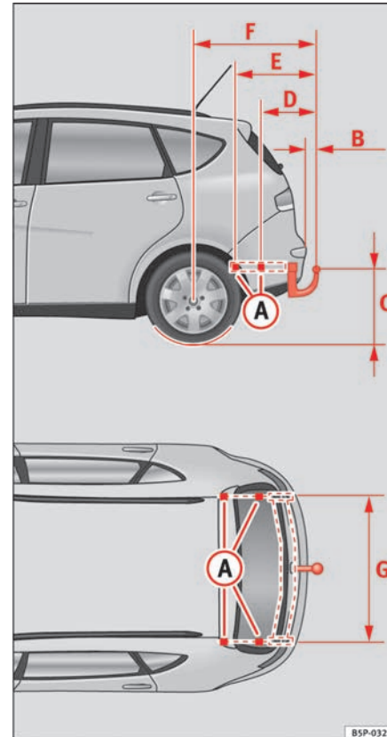
Abb. 160 Befestigungspunkte für die Anhängervorrichtung
