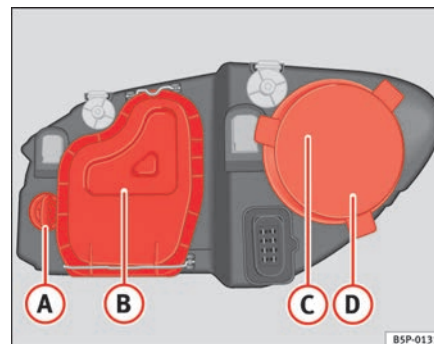
Abb. 185 Glühlampen des Hauptscheinwerfers
