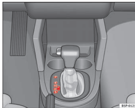
Abb. 140 Ausschnitt aus der Mittelkonsole: Wählhebel vom Automatikgetriebe / Direktschaltgetriebe DSG
