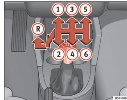
Abb. 139 Ausschnitt aus der Mittelkonsole: Schalt-schema vom 6-Gang-Schaltgetriebe
