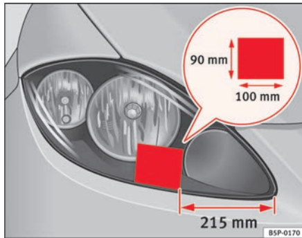
Abb. 156 Rechter Scheinwerfer
