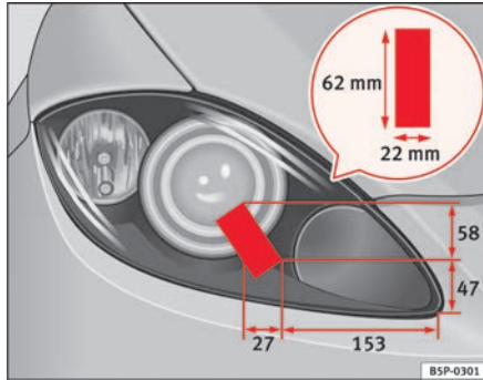
Abb. 158 Rechter Scheinwerfer
