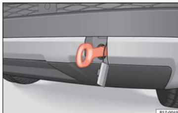
Abb. 78 Hinterer Stoßfänger rechts: Eingeschraubte Abschleppöse
