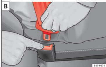
Abb. 93 Schlosszunge des Sicherheitsgurts in das Gurtschloss einstecken und vom Gurtschloss lösen.
