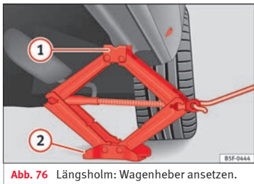
Abb. 76 Längsholm: Wagenheber ansetzen.
