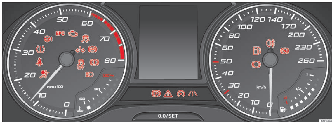
Abb. 51 Display des Kombi-Instruments in der Instrumententafel.
