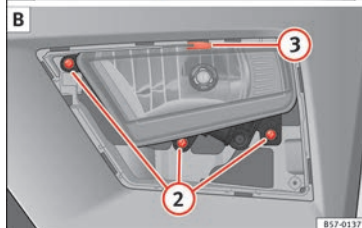
Abb. 109 Nebelscheinwerfer: Blende herausziehen.
