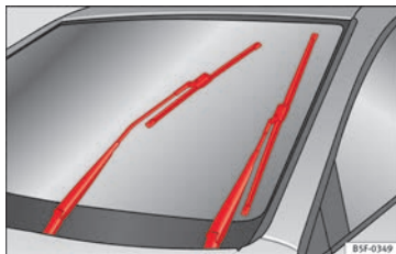
Abb. 81 Scheibenwischer in Servicestellung.
