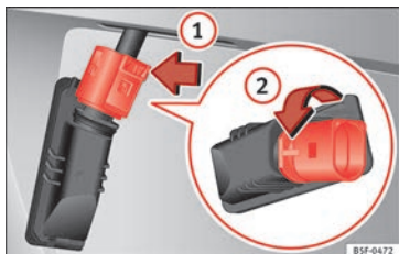
Abb. 116 Kennzeichenleuchte: Lampenträger ausbauen.
