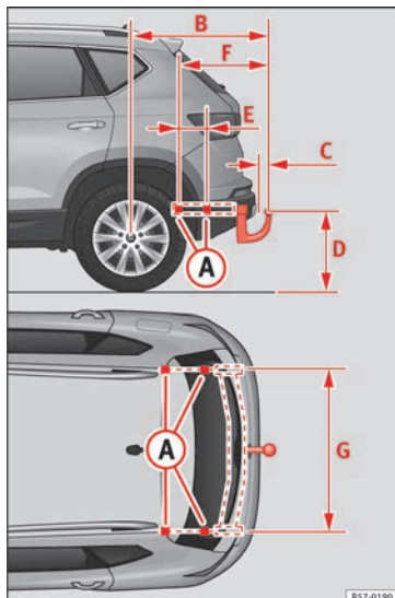
Abb. 237 Maße und Befestigungspunkte für den nachträglichen Einbau einer Anhängervorrichtung
