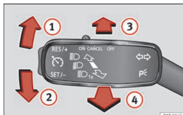
Abb. 37 Blinker- und Fernlichthebel.
