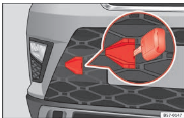
Abb. 98 Auf der rechten Seite des vorderen Stoßfängers: Abdeckung entfernen.
