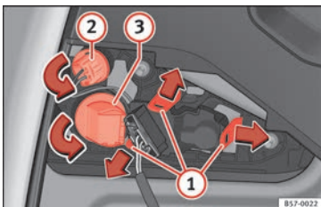
Abb. 114 Lampenhalter ausbauen.
