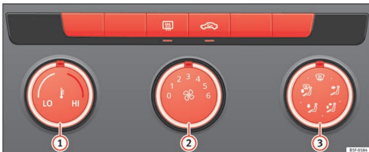
Abb. 59 Mittelkonsole: Systembedienungen für Heiz- und Frischluft
