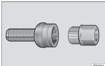
Abb. 73 Diebstahlhemmende Radschraube mit Abdeckkappe und Adapter
