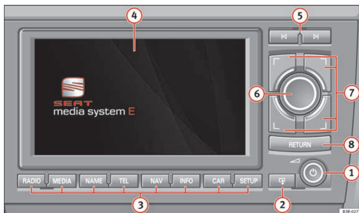
Abb. 1 Bedieneinheit des Navigationssystems SEAT Media System
