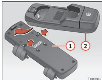
Abb. 85 Mobiltelefon-Adapter einbauen
