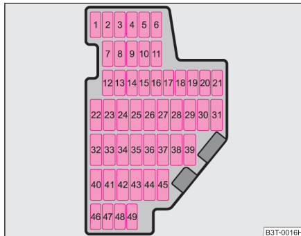
Abb. 216 Schematische Darstellung des Sicherungsträgers in der Schalttafel
