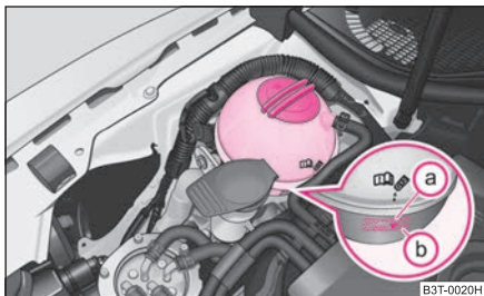
Abb. 189 Motorraum: Kühlmittel-Ausgleichbehälter
