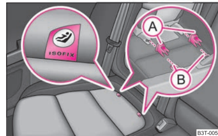
Abb. 172 Halteösen (ISOFIX-System)
