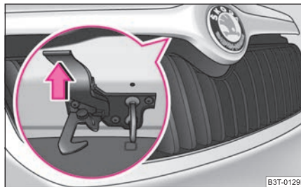
Abb. 186 Kühlergrill: Zugriff
