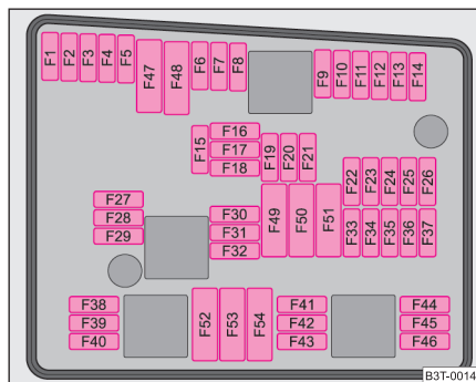
Abb. 214 Schematische Darstellung der Sicherungsbox im Motorraum - Ausführung 1
