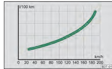
Abb. 166 Kraftstoffverbrauch in l/100 km und Geschwindigkeit in km/h
