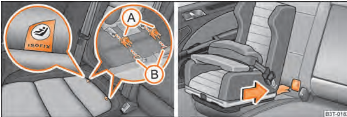
Abb. 159 Halteösen (ISOFIX-System) / der ISOFIX-Kindersitz wird in die montierten Aufnahmebohrer geschoben
