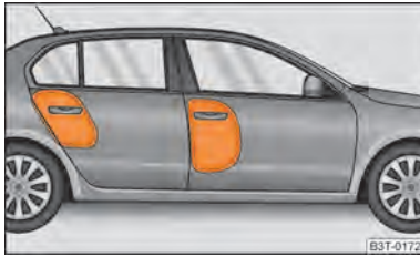
Abb. 149 Gasgefüllte Seiten-Airbags
