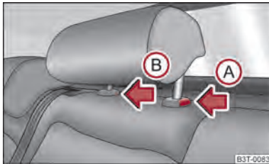
Abb. 60 Rücksitze: mittlere Kopfstütze
