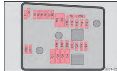
Abb. 201 Schematische Darstellung der Sicherungsbox im Motorraum - Ausführung 2
