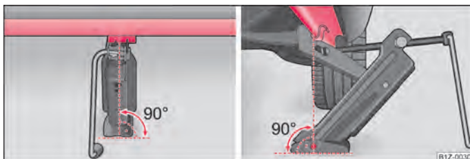
Abb. 190 Wagenheber ansetzen
