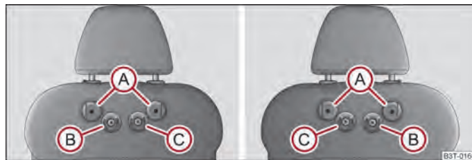
Abb. 137 Sitzlehne - linker Vordersitz / rechter Vordersitz
