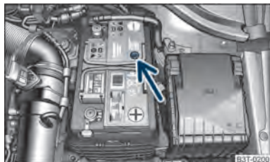
Abb. 177 Batterie: Anzeige Elektrolytstand
