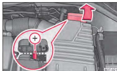
Abb. 195 Detail des Motorraums: Starthilfepunkt
