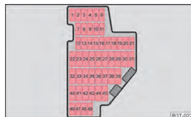
Abb. 202 Schematische Darstellung des Sicherungsträgers in der Schalttafel
