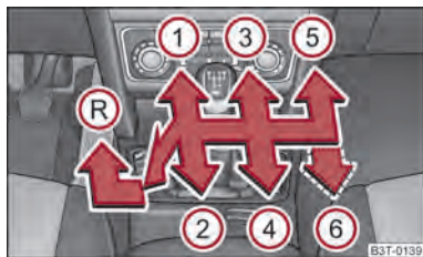
Abb. 116 Schaltschema: 5-Gang bzw. 6-Gang Schaltgetriebe
