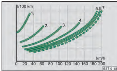
Abb. 165 Kraftstoffverbrauch in l/100 km und Geschwindigkeit in km/h
