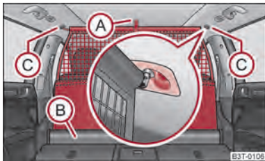
Abb. 83 Gepäcknetztrennwand herausziehen
