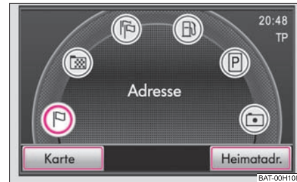
Abb. 13 Hauptmenü Navigation
