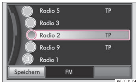
Abb. 6 FM-Senderliste
